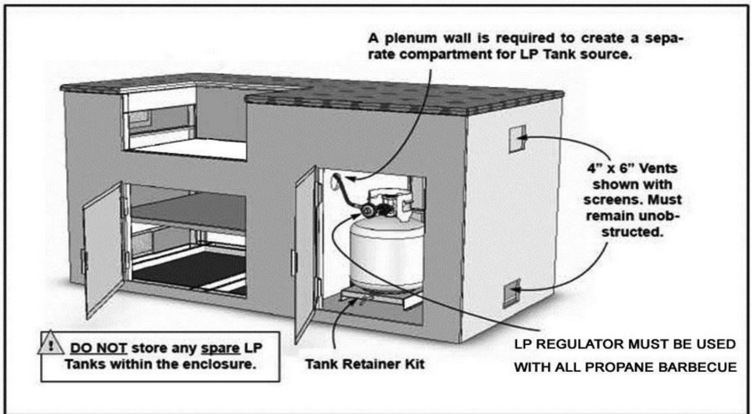
Méthode d'installation pour le gaz à basse pression
